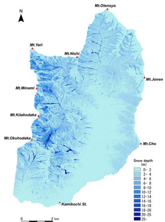
図1. 上高地梓川流域における積雪深分布
